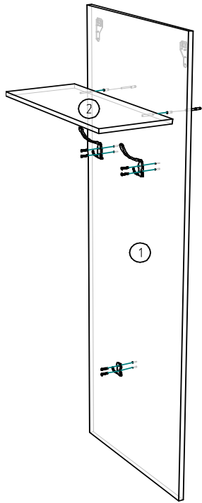
Схема сборки вешалки (рис.1)
