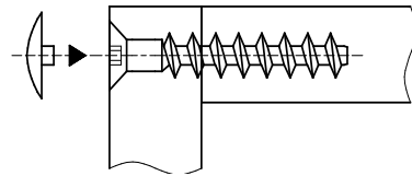
Схема крепления евровинтов (рис.3)
