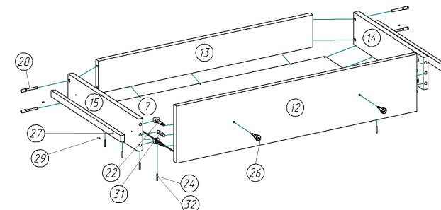
Рис.5 Сборка ящиков
