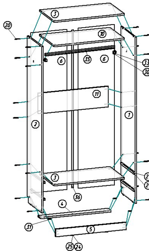
Рис.1 Сборка корпуса
