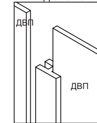
Схема крепления соедин.элемента
